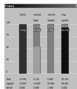
电源消耗图
